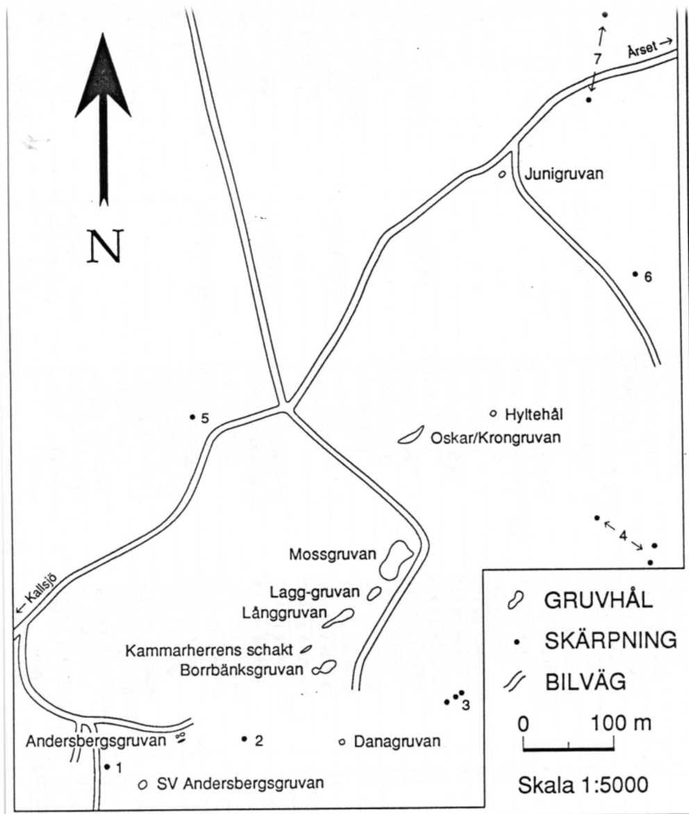
Fig. 5. Fredriksbergs gruvfält. Siffrorna vid skärpningarna anger skärpningens namn eller motsvarande utmåls namn.
